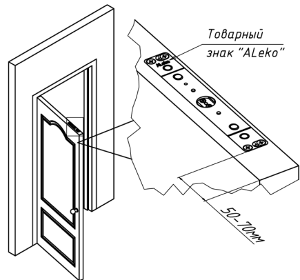
Рисунок 3 – Установка замка в горизонтальном варианте
